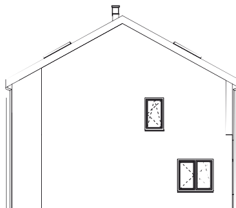
elewacja boczna prawa
