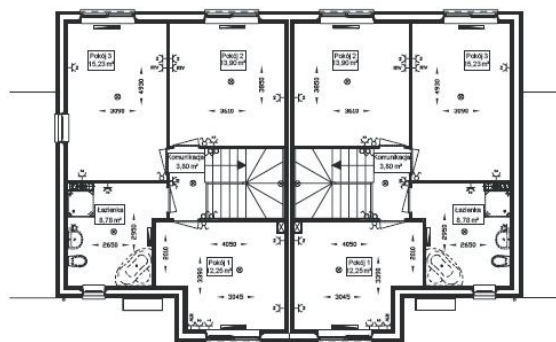
piętro
